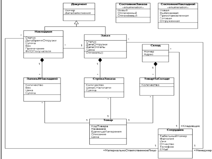
Рис. 2 Диаграмма UML
