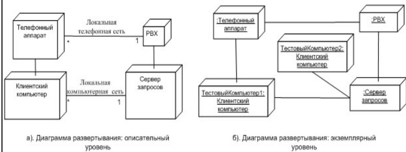
Рис. 3 Диаграмма UML
