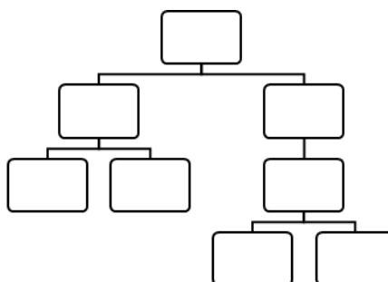
Рисунок 5. Иерархическая структура
