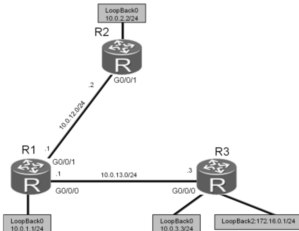
Рис. 4.4 Топология OSPF для одной зоны
