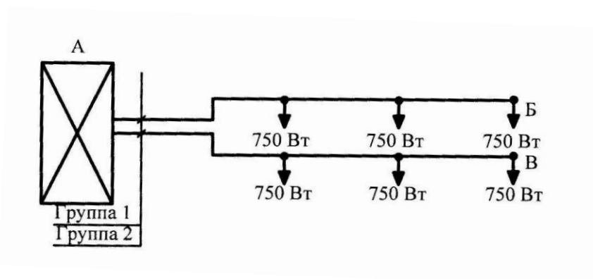
Рисунок 1.3 - Расчетная схема
