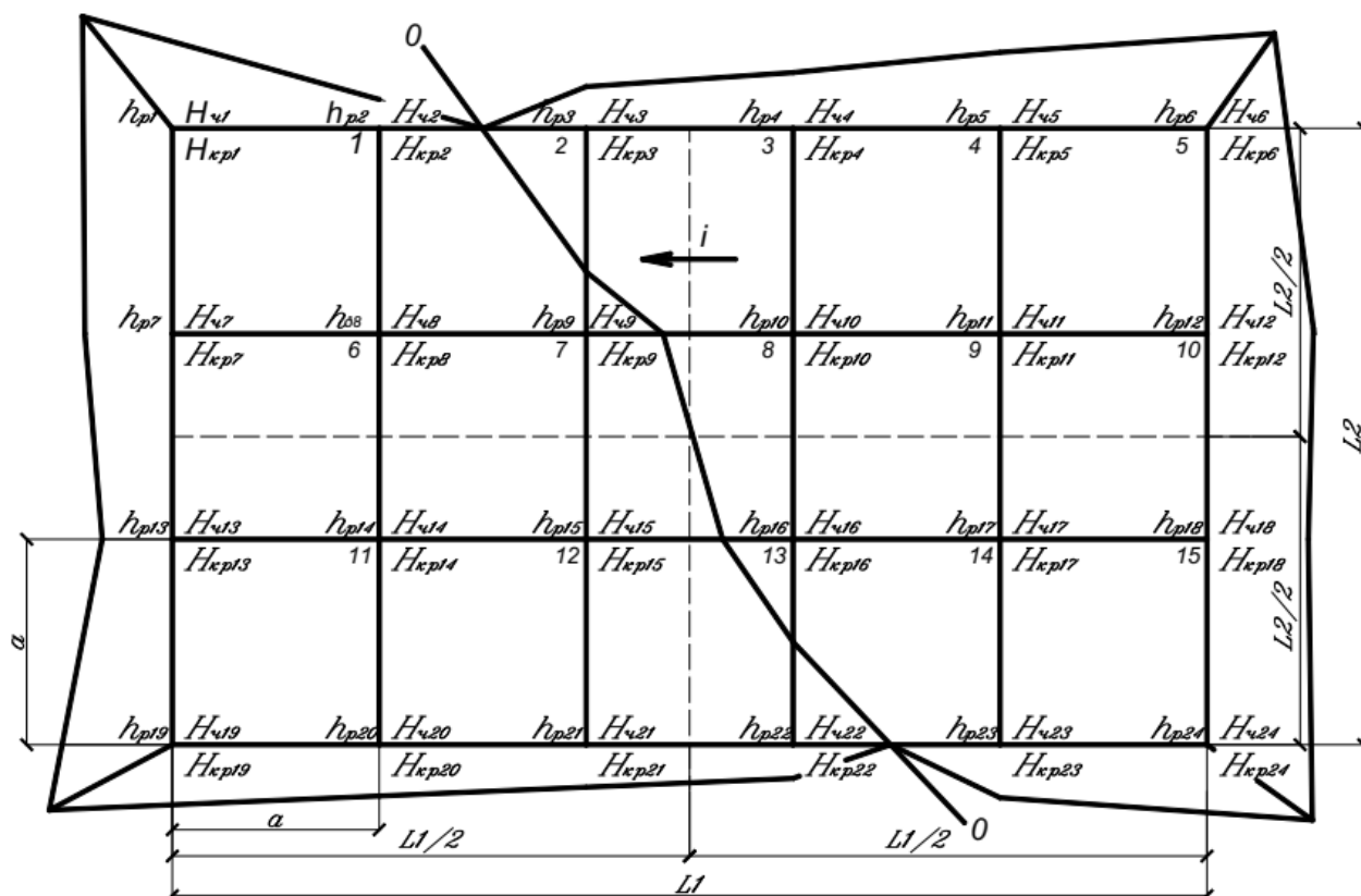
Рисунок П.2 – План площадки с нанесением черных, красных, рабочих отметок и линии нулевых работ
