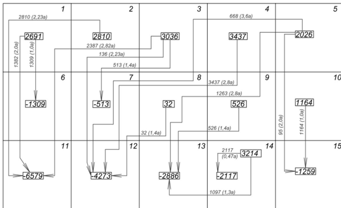
Рисунок П.3 - Картограмма земляных масс
