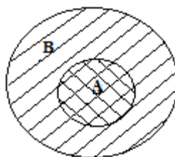
Рис. 14 A \cap B = A .
