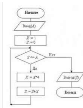
Рис.1. Блок-схема алгоритма
