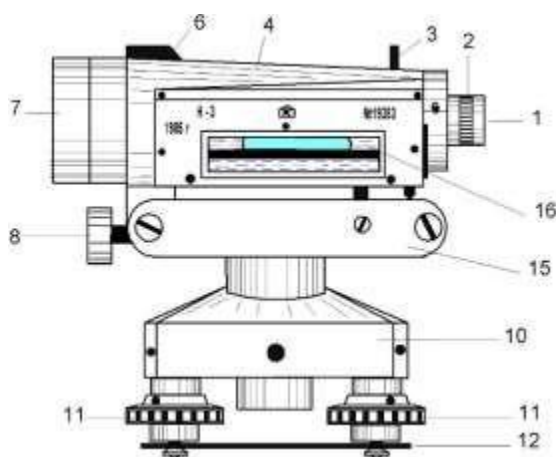
Рис. 1. Нивелир НЗ:
