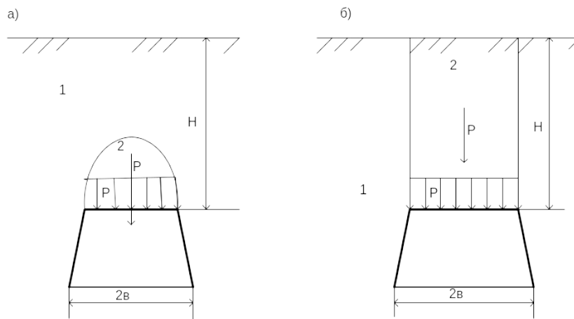
Рис. 1. Расчетная схема к определению на крепь в соответствии с моделью: а – М.М. Протодьяконова; б – опускающегося столба; 1 – жесткая область; 2 – пластическая область.
