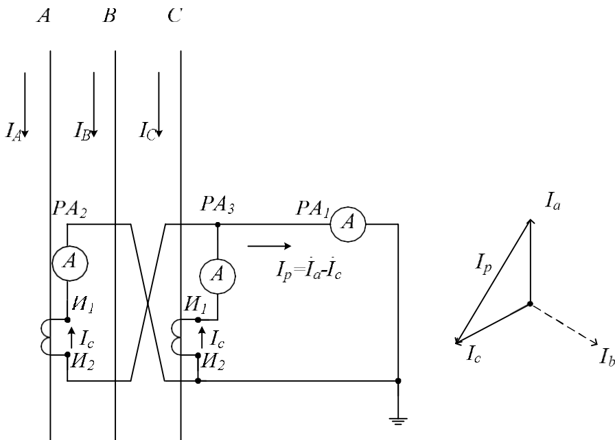
Рис. 3. Схема соединения трансформаторов тока на разность токов двух фаз
