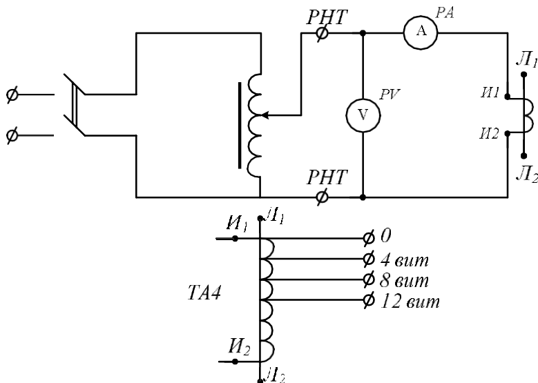
Рис.13. Схема снятия характеристики намагничивания трансформатора тока.
