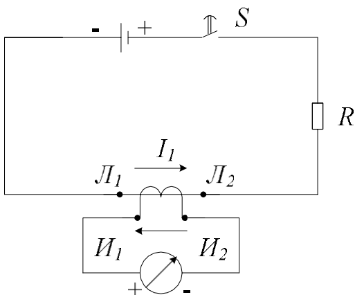
Рис.6. Схема проверки полярности обмоток трансформатора тока
