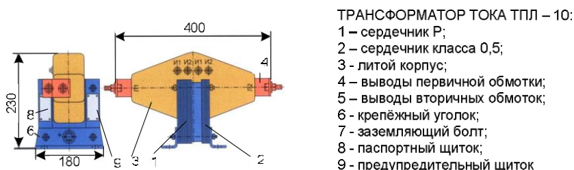
Рис.5. Внешний вид и разрез одновиткового трансформатора тока ТПЛ-10 В
