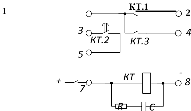
Рис.3. Реле времени серии ЭВ-100 с искрогасительным контуром
