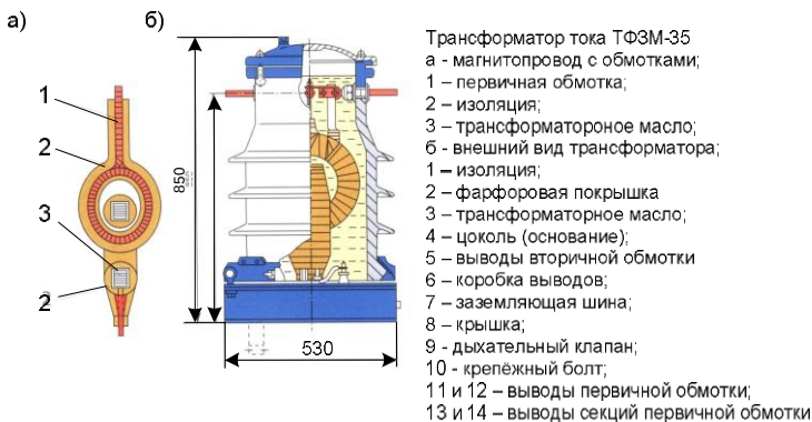
Рис.3. Внешний вид и разрез однокаскадный трансформатора тока ТФЗМ - 35
