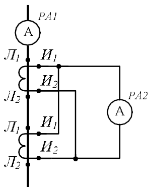
Рис.9. Схема параллельного включения двух трансформаторов тока на одной фазе
