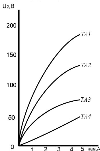
Рис. 12. Характеристики намагничивания
