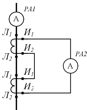
Рис.8. Схема последовательного включения двух трансформаторов тока на одной фазе
