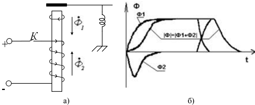
Рис.1. Влияние короткозамкнутой обмотки на работу реле при его включении и выключении
