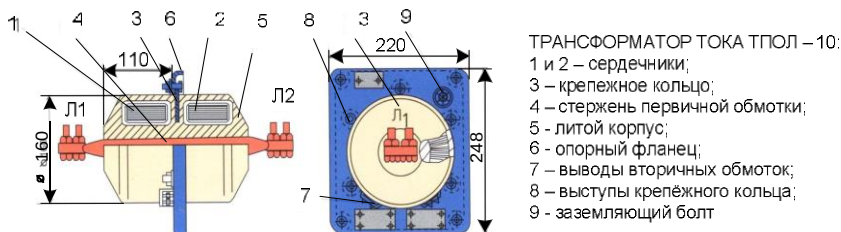
Рис.4. Внешний вид и разрез одновиткового трансформатора тока ТПОЛ-10
