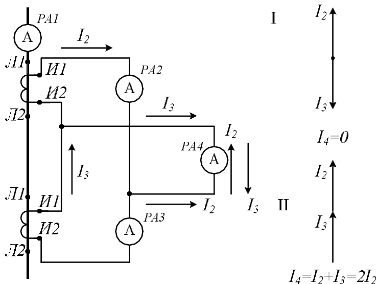
Рис..11. Схема включения трансформаторов тока по дифференциальной схеме
