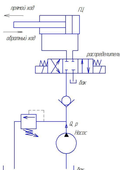
Рисунок 1 – Гидравлические схемы подключения гидроцилиндра
