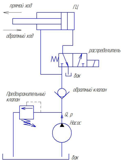
Рисунок 1 – Гидравлические схемы подключения гидроцилиндра
