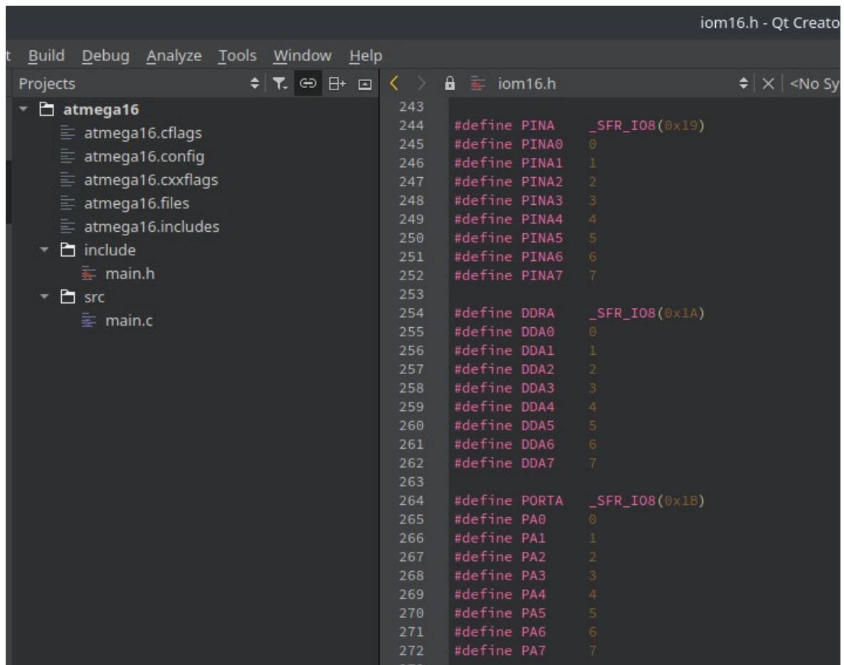
Рис. 21.2. Описание периферии контроллера
