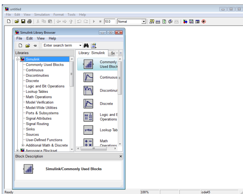
Рис. 1.5. Библиотека MATLAB
