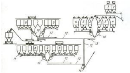
Рис. 6. Схема шихтоподати доменной печи "Amalinda" объемом 2032 м³: 1 - бункера окатышей; 2,3 - бункера известняка; 4 - бункера агломерата и руды; 5 - бункера окатышей и руды; 6,7 - бункера мела; 8 - бункера доменного газа; 9 - бункер скрапа; 10 - весовые воронки; 11-13 - питательные веса; 14 - скип
