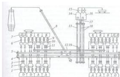
Рис. 5.70. Схема конвейерной шихтоподати доменной печи объемом 5000 м³
