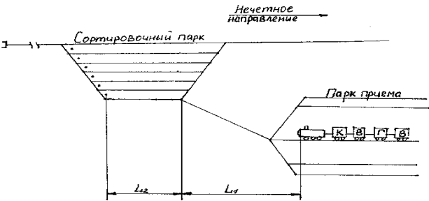
Рис. 1.1 Фрагмент путевого развития станции А
