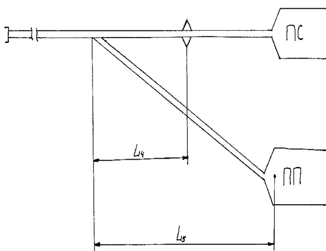
Рисунок 4 – Вариант взаимного расположения парков (для выполнения задания 2).
