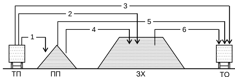
Рис. Принципиальная технологическая схема переработки груза в транспортно-грузовом комплексе
