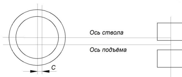
Рис.4.1. Геометрическая схема подъемного комплекса
