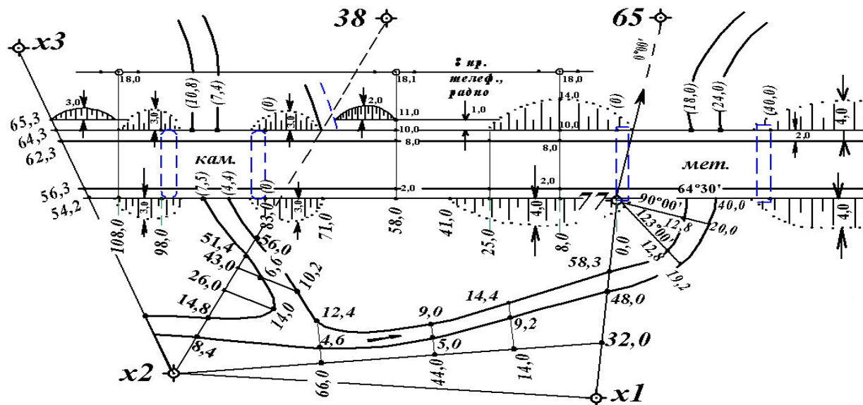
Рис. 11. Абрис теодолитной съёмки
