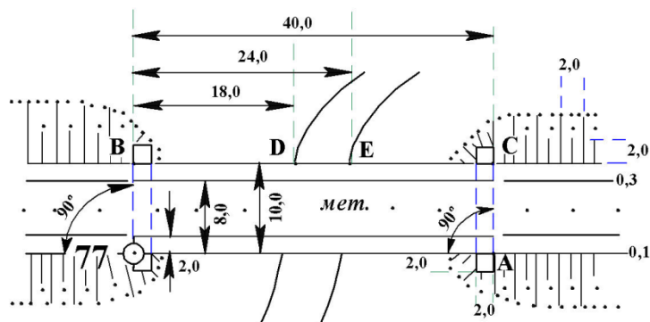
Рис. 14. Построение металлического моста и береговых линий
