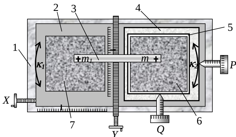
Рис. 8.6 Схема стереокомпа-
