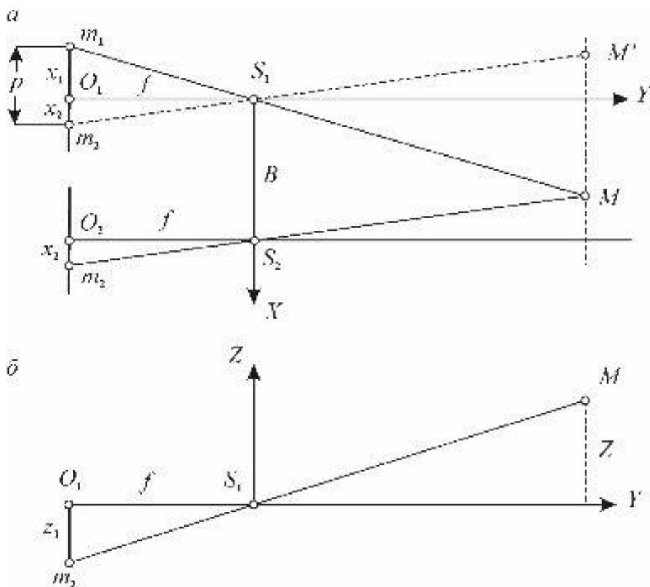
Рис. 1.4 Связь координат x, z на снимках
