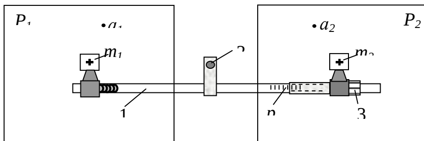
Рис. 51. Параллаксометр
