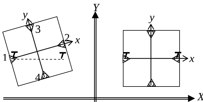
Рис. 8.8 Ориентирование снимков по координатным меткам
