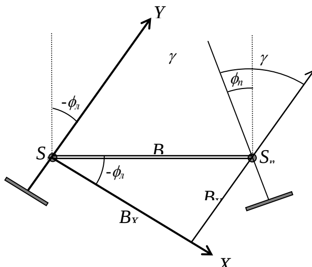
Рис. 1.5 конвергентная съемка
