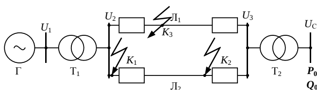
Рисунок. Расчетная схема
