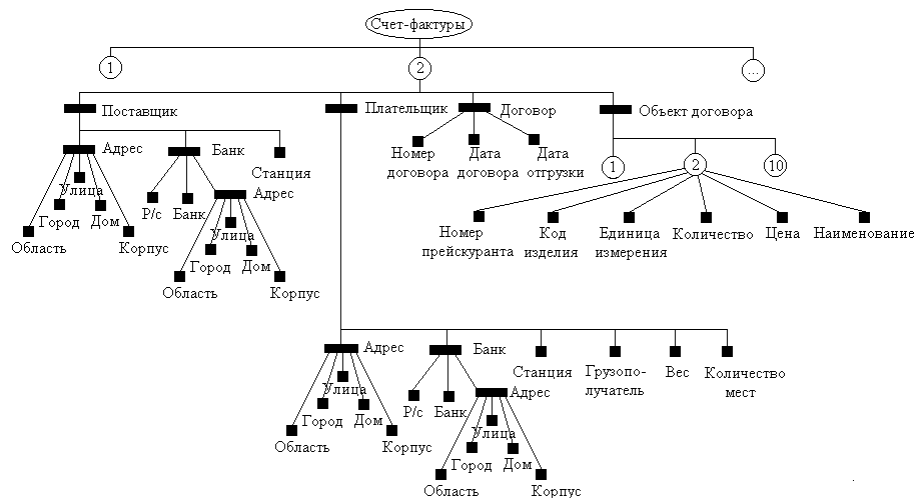
Рис. 4.5. Структура составной единицы информации для счет-фактуры Задача 4.3
