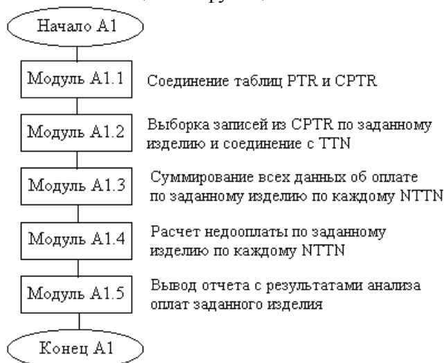
Рис. 5.5. Блок-схема решения подзадачи А1
