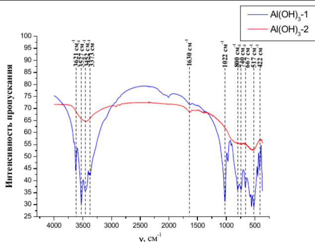
Рис.4.1. ИК спектры гидроксида алюминия Al(OH) 3 -1 и вещества, которое было получено после проведения термogravиметрического анализа Al(OH) 3 -1 (обозн. Al(OH) 3 -2). Спектры сняты с таблеток в КВТ.
