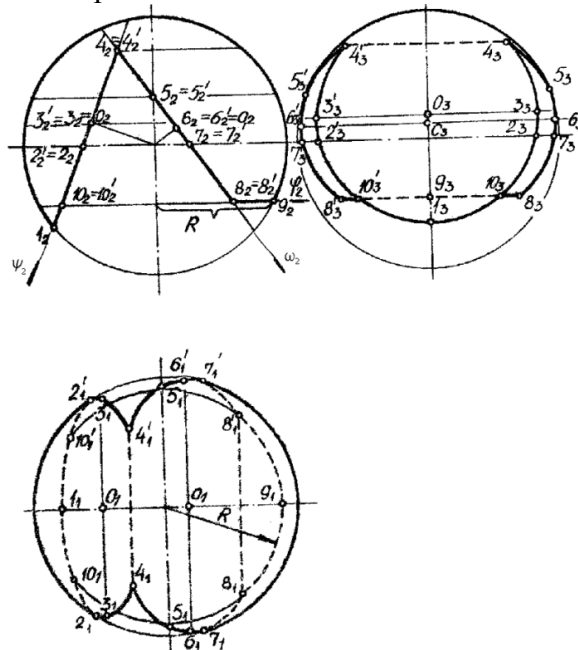
Рис.2. Сфера с вырезом ( пересечение поверхности вращения плоскостями)
