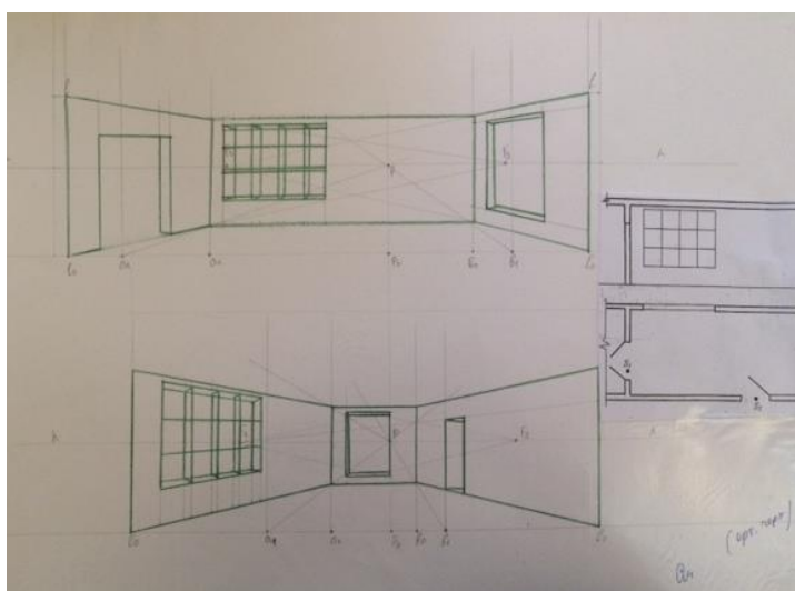
Рис.6. Построение перспективы интерьера методом широкоугольной перспективы
