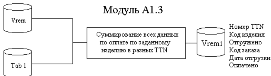
Рис. 5.10. Функционально-технологическая схема модуля А1.3
