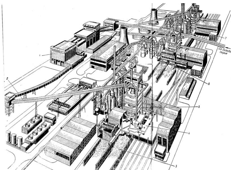
Рис. III.7. Устройство доменного цеха с отделением прокатки брусков и ковалей из расплавленной стали «Южсталь» (Франция): 1 — отделение прокатки брусков и ковалей; 2 — ковалевая система; 3 — шихтовый ящик; 4 — литейный ящик; 5 — доменная печь; 6 — система газоочистки; 7 — воздухоподогреватель
