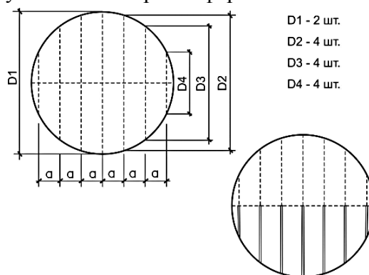
Рисунок 17. Развертка сферы с 6 сегментами
