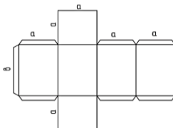
Рисунок 6. Развертка квадратной призмы
