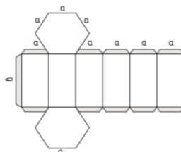
Рисунок 8. Развертка правильной шестиугольной призмы
