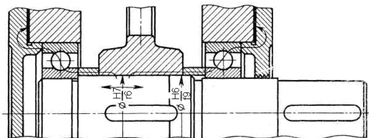
4. Узел выходного вала
