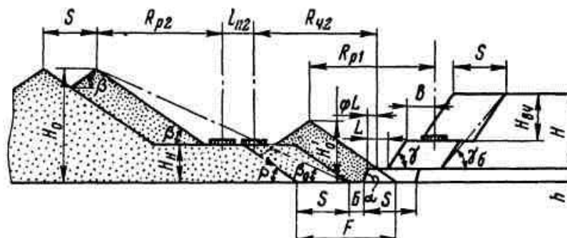
Рис. 1 Схема экскавации с драглайнами на вскрышном подуровне
