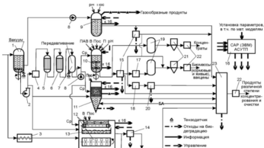
Рисунок 1 – Принципиальная схема реализации биотехнологических процессов (по У. Э. Виестур и др.):
