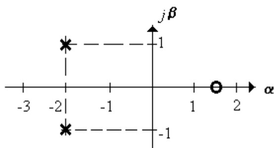
№8. Записать передаточную функцию системы с картой нулей-полюсов (рисунок 1.10) и общим коэффициентом передачи k = 1,2 (кратных корней нет).
