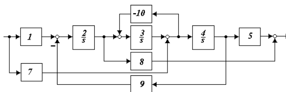
№7. Определить передаточную функцию схемы (рисунок 1.9)
