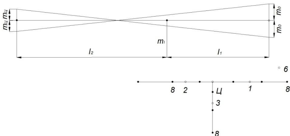
Рис. 2.2 Рекогносцировочная схема
